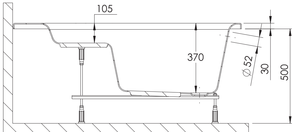
PRZEKRÓJ A-A
