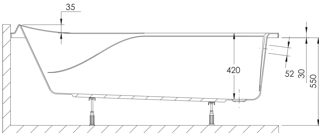
PRZEKRÓJ A-A
