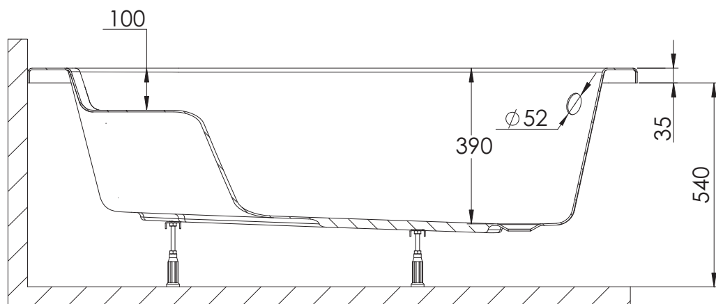
PRZEKRÓJ A-A
