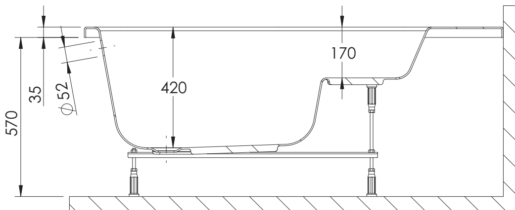
PRZEKRÓJ A-A
