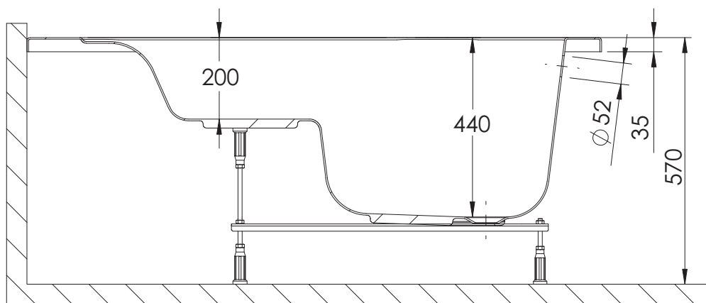
PRZEKRÓJ A-A
