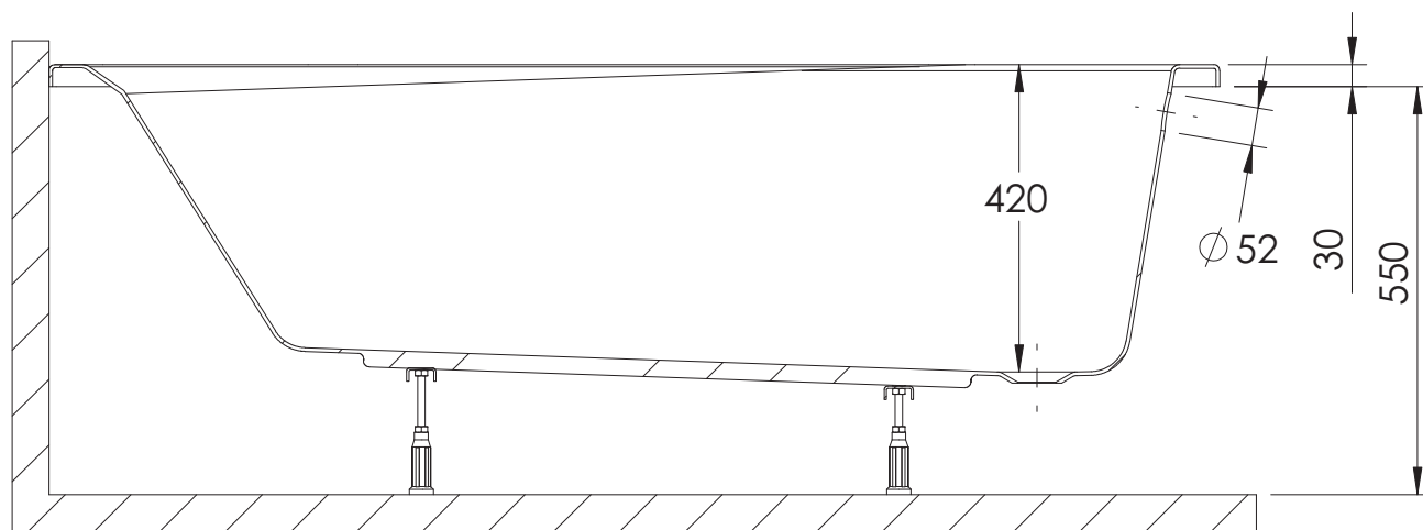
PRZEKRÓJ A-A
